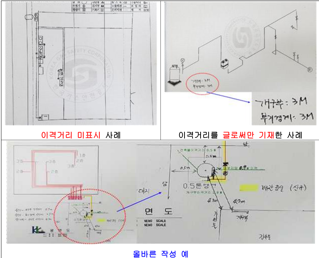
[ 그림 ] 소형저장탱크 이격거리 표시 도면 징구 부적정 예시
